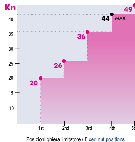
Posizioni ghiera limitatore / Fixed nut positions
