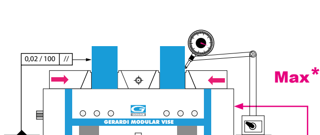
Morsa ancorata con 2 coppie di staffe Art.296 Vise clamped with n. 2 pairs of Art.296
